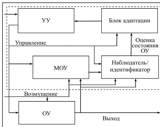
Рис. 4. Структура адаптивной системы автоматического управления с наблюдателем/идентификатором
